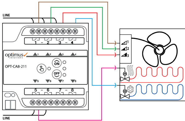
3-Hızlı Fan Coil, 2x Aç/Kapa Vana
