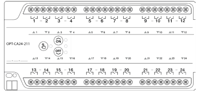
Kombine Aktuatör 24 kanal
