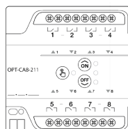
Kombine Aktuatör 8 kanal
